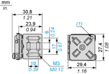
(1) 2 screws M3 x 12
