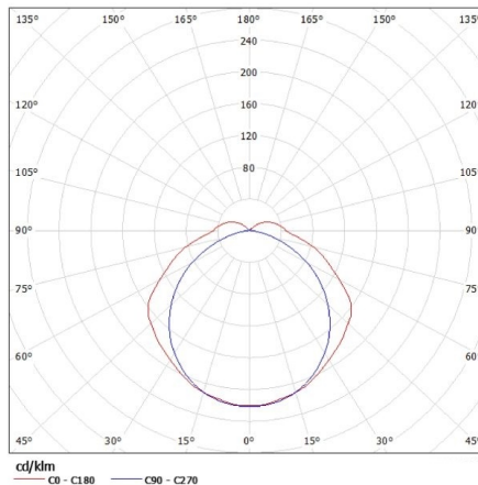
KANLUX S.A. (kat 18519) MAH PLUS-136 - T8 LED SMD / Krzywa rozsyłu światła (biegunowo)
