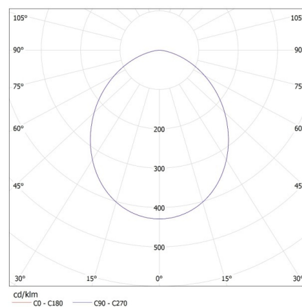
KANLUX S.A. (kat 25510) TIBERI LED SMD 24W / Krzywa rozsyłu światła (biegunowo)
