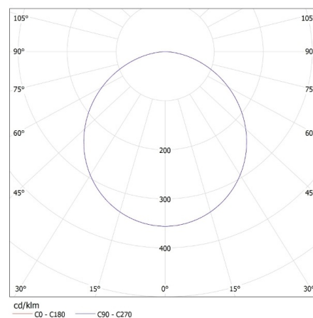
MILED (kat 31075) SP LED N 6W NW-S / LDC (Polar)
