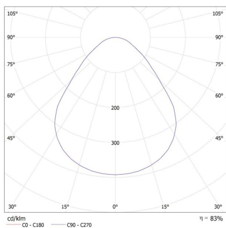
KANLUX S.A. (kat 29818) BLINGO RU 36W 6060 NW / LDC (Polar)
