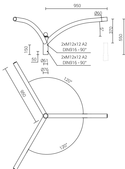
Kod Nazwa Przeznaczenie Ilość ramion Objętość jednostkowa Powierzchnia boczna Średnica montażowa oprawy Waga netto 472023/C... WR-2/3/0,95/5 słupy aluminiowe z zakończeniem ø60x180 3 0.26 m³ 0.145 m² ø60 mm x 100 mm 6.3 kg
