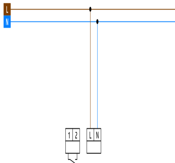
Schemat połączeń
