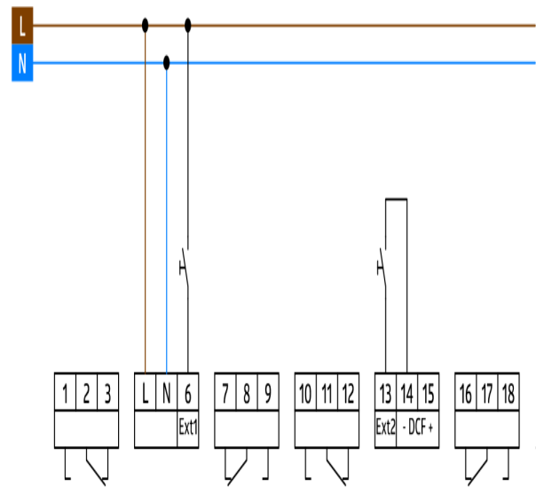
Schemat połączeń
