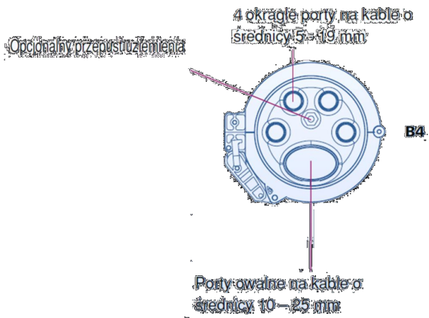
FOSC 400 B4 - Konfiguracja portów kablowych
