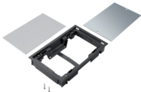
tehalit.VE-EE Pokrywa pełna płytki montaż E04 147X247 5mm czarny PA
