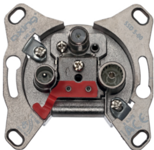
tehalit.WA Mechanizm gniazda RTV-SAT pojedynczego-końcowego 0dB 5-2200MHz
