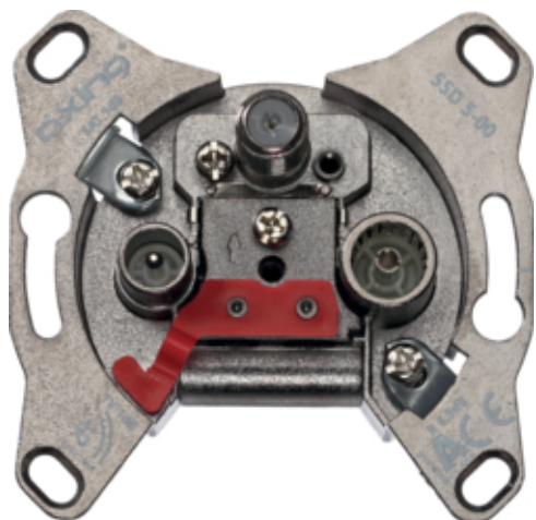
tehalit.WA Mechanizm gniazda RTV-SAT końcowego 7dB 5-2200MHz
