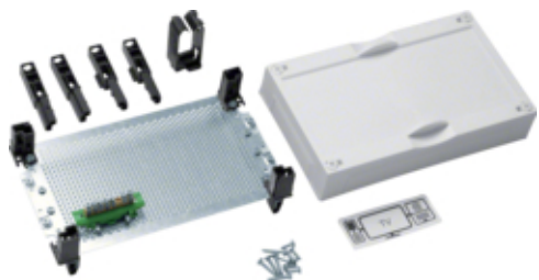
univers N Podzespół 150x250mm do VDI
