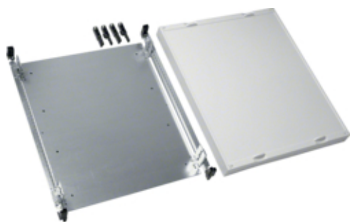
univers N Blok z płytą montażową 600x500mm
