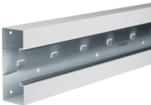
tehalit.BRS Podstawa 170mm, stalowa, biała
