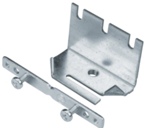
tehalit.BK Wspornik poziomy do kanałów BK AB wys. 65mm stal
