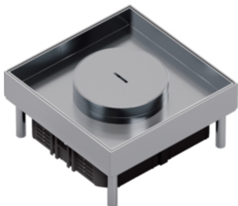
tehalit.VE-EE Pokrywa tubus IP54 20kN EKSQ06 200X200 25mm stal nierdzewna
