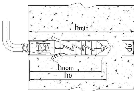
Parametry montażu dla wkrętów z hakiem kątowym
