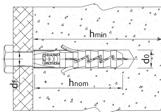
Parametry montażu
