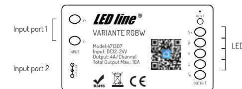
Rys.1 Widok kontrolera
