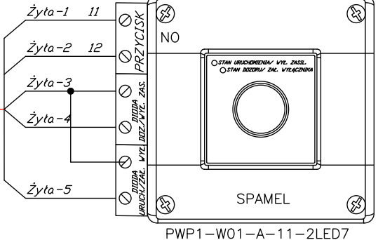
DETAL A PWP URZĄDZENIE URUCHAMIAJĄCE
