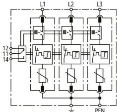
Schemat połączeń DG M TNC ACI 275 FM
