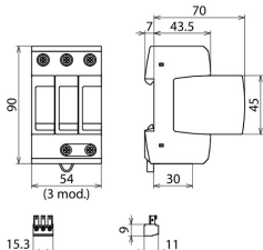
Rysunek wymiarowy DG M TNC ACI 275 FM
