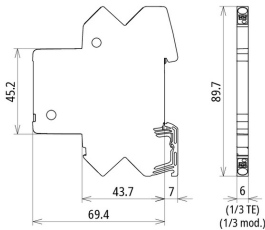
Rysunek wymiarowy BCO CL2 BD EX 24
