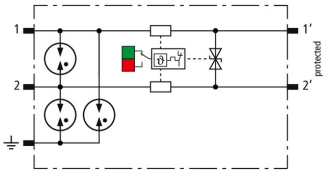
Schemat połączeń BCO CL2 BD EX 24
