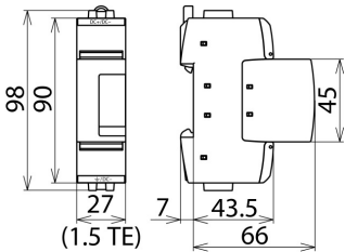
Rysunek wymiarowy DG SE DC 60
