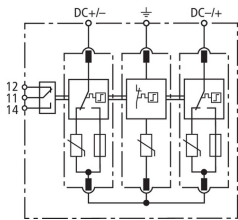
Schemat połączeń DG M YPV SCI 150 FM
