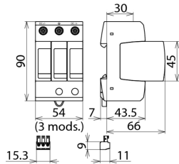
Rysunek wymiarowy DG M YPV SCI 150 FM
