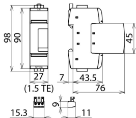
Rysunek wymiarowy DG SE CI WE 440 FM
