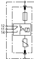
Schemat połączeń DG SE CI WE 440 FM
