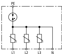
Schemat połączeń DG TT 5 275
