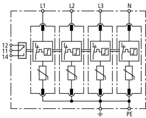
Schemat połączeń DG M TNS 275 FM
