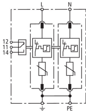
Schemat połączeń DG M TN 150 FM
