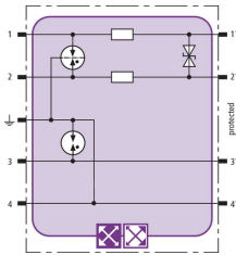
Schemat połączeń BXT ML2 BD S 24 48
