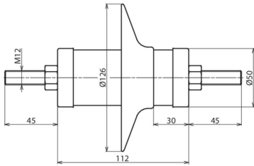
Rysunek wymiarowy DMI 6 10 1 N
