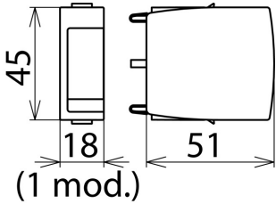
Rysunek wymiarowy DG MOD 48
