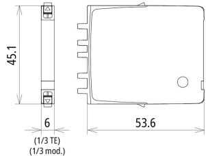
Rysunek wymiarowy BCO MOD ML2 BE HF 24
