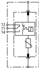
Schemat połączeń DG S 48 FM
