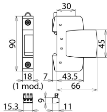
Rysunek wymiarowy DG S 75 FM
