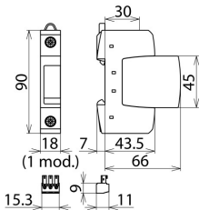
Rysunek wymiarowy DG S WE 600 FM
