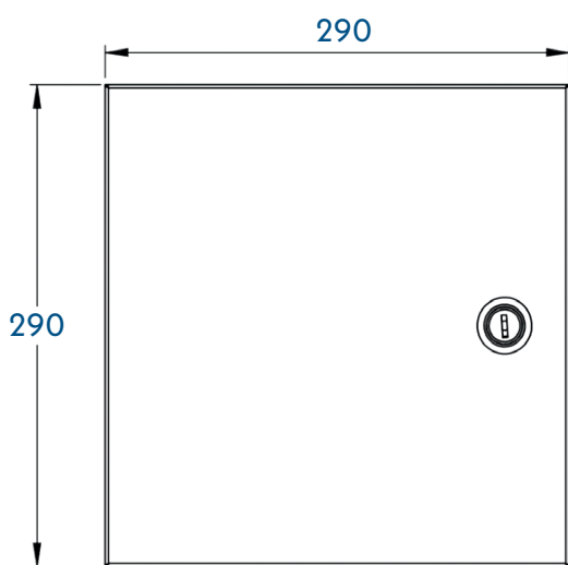
WIDOK PRZODU
