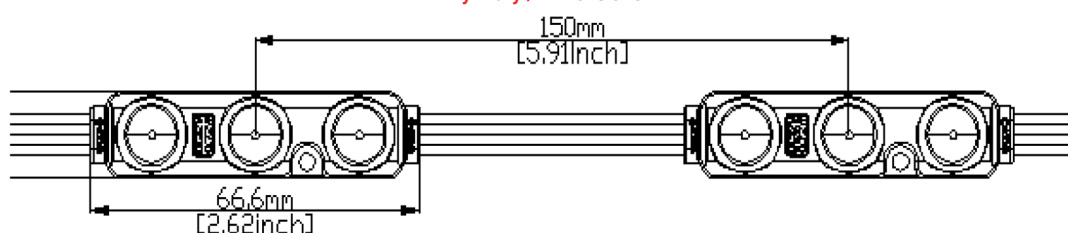
Wymiary / Dimensions
