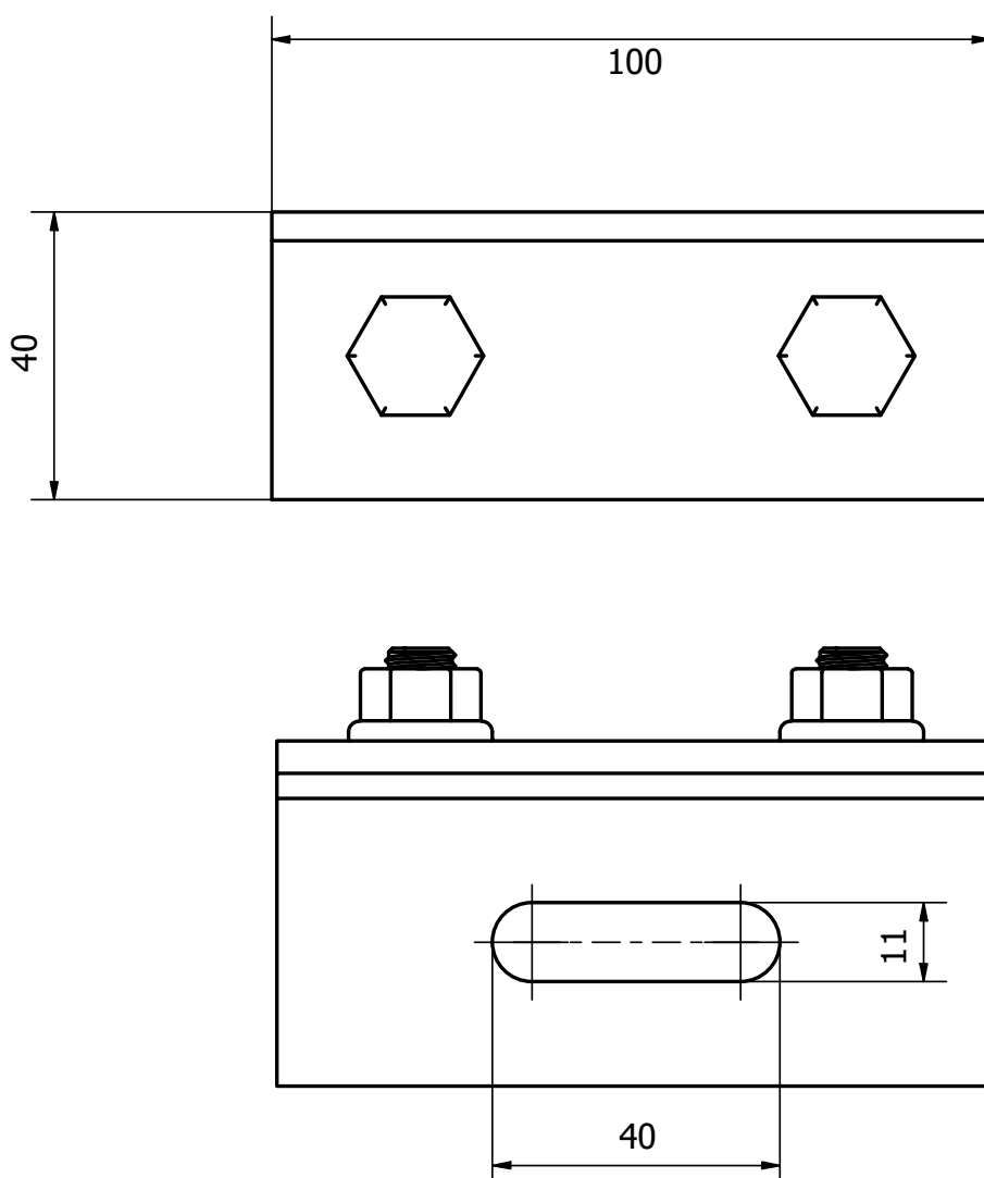
Rys.1 Wymiary uchwytu K-24-Z
