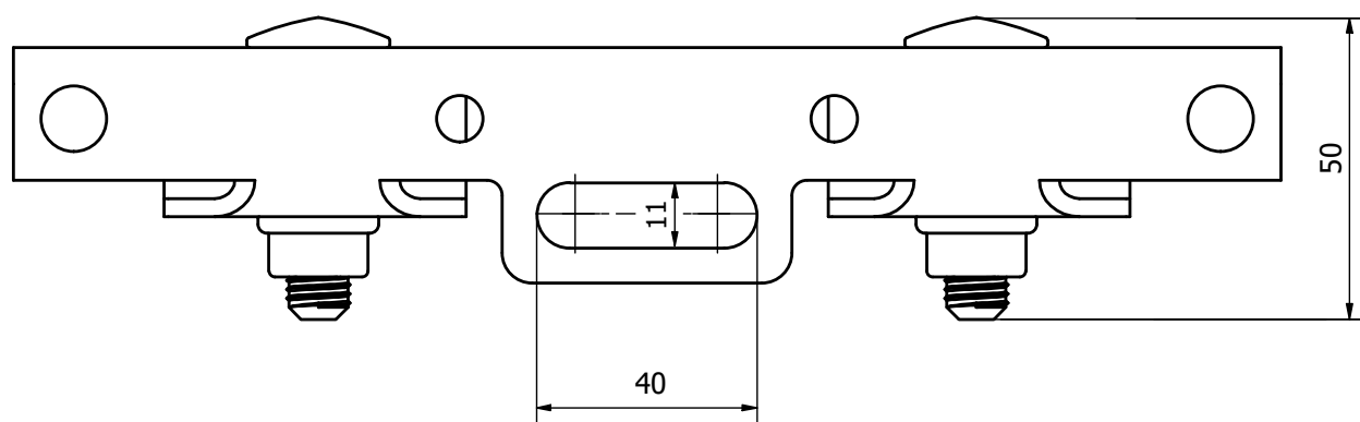
Rys.2 Wymiary uchwyty K-24-C
