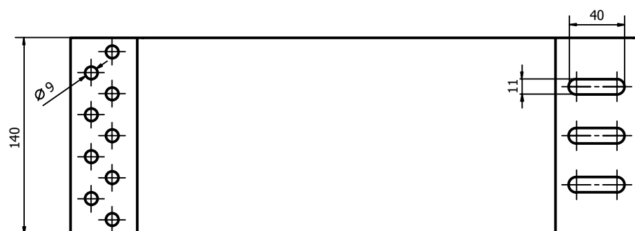
Rys.3 Wymiary elementu K-44-W - rzut od góry
