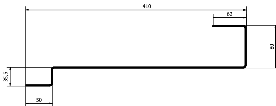
Rys.3 Wymiary elementu K-44-W - rzut od boku
