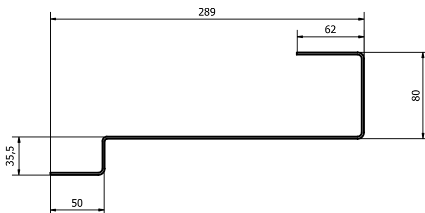
Rys.1 Wymiary elementu K-44 - rzut od boku.
