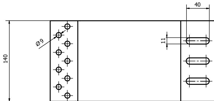
Rys.2 Wymiary elementu K-44 - rzut od góry.
