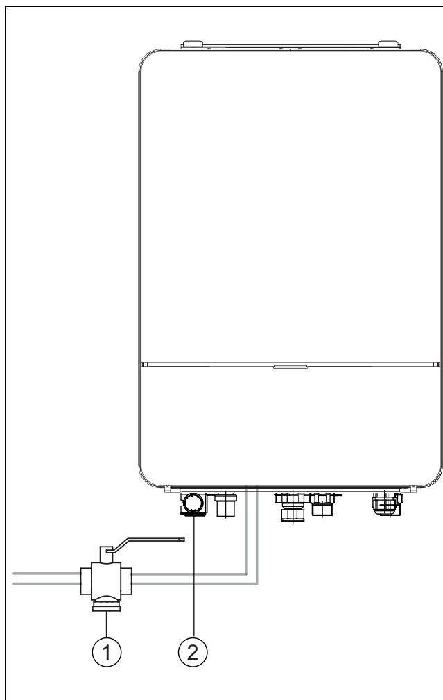
Rys. 7 Jednostka wewnętrzna AWB
