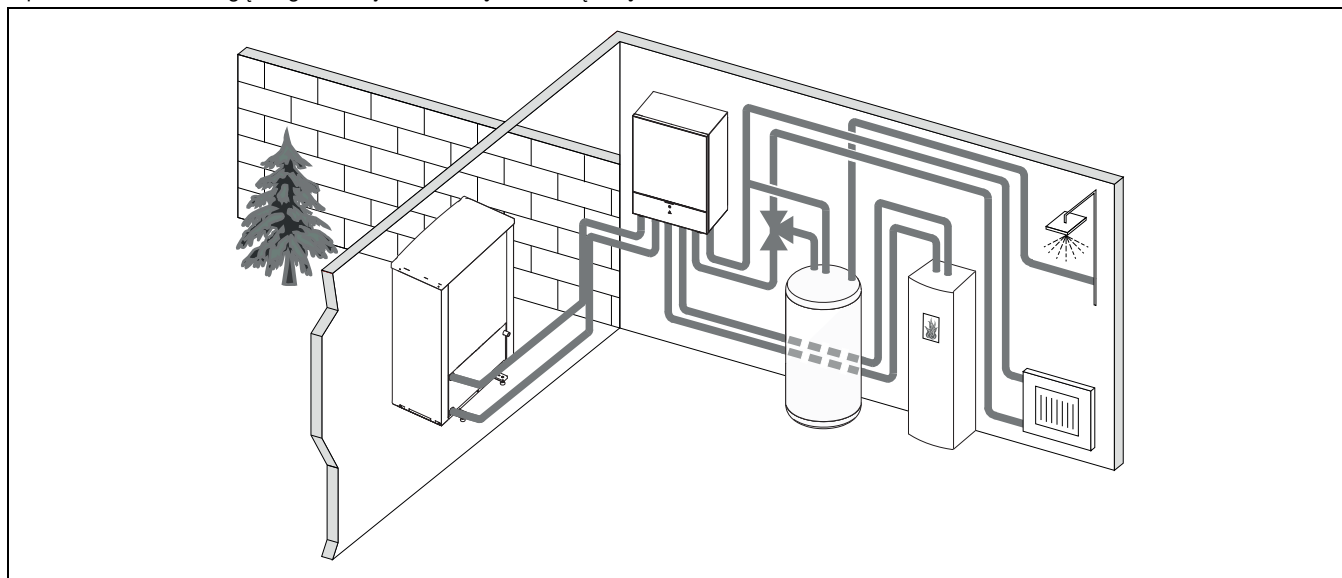
Rys. 3 Pompa ciepła Compress 7000i AW, jednostka wewnętrzna AWB bez dogrzewacza elektrycznego, zewnętrzny podgrzewacz pojemnościowy c.w.u. i zewnętrzny dogrzewacz
