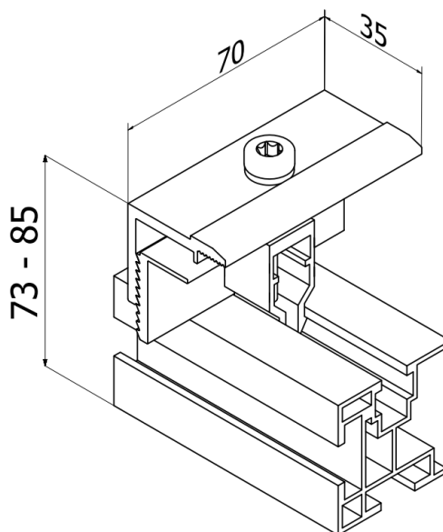
Rys.2 Wymiary elementu K-06-R
