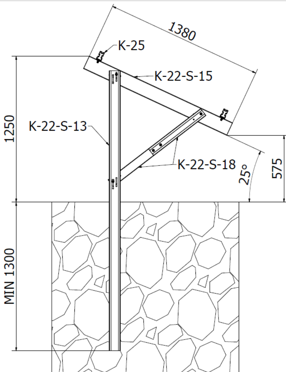
Rys.1 Wymiary konstrukcji
