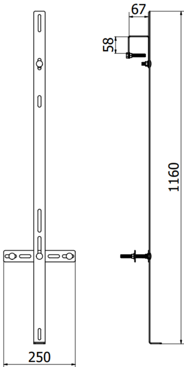
Rys.1 Wymiary konstrukcji
