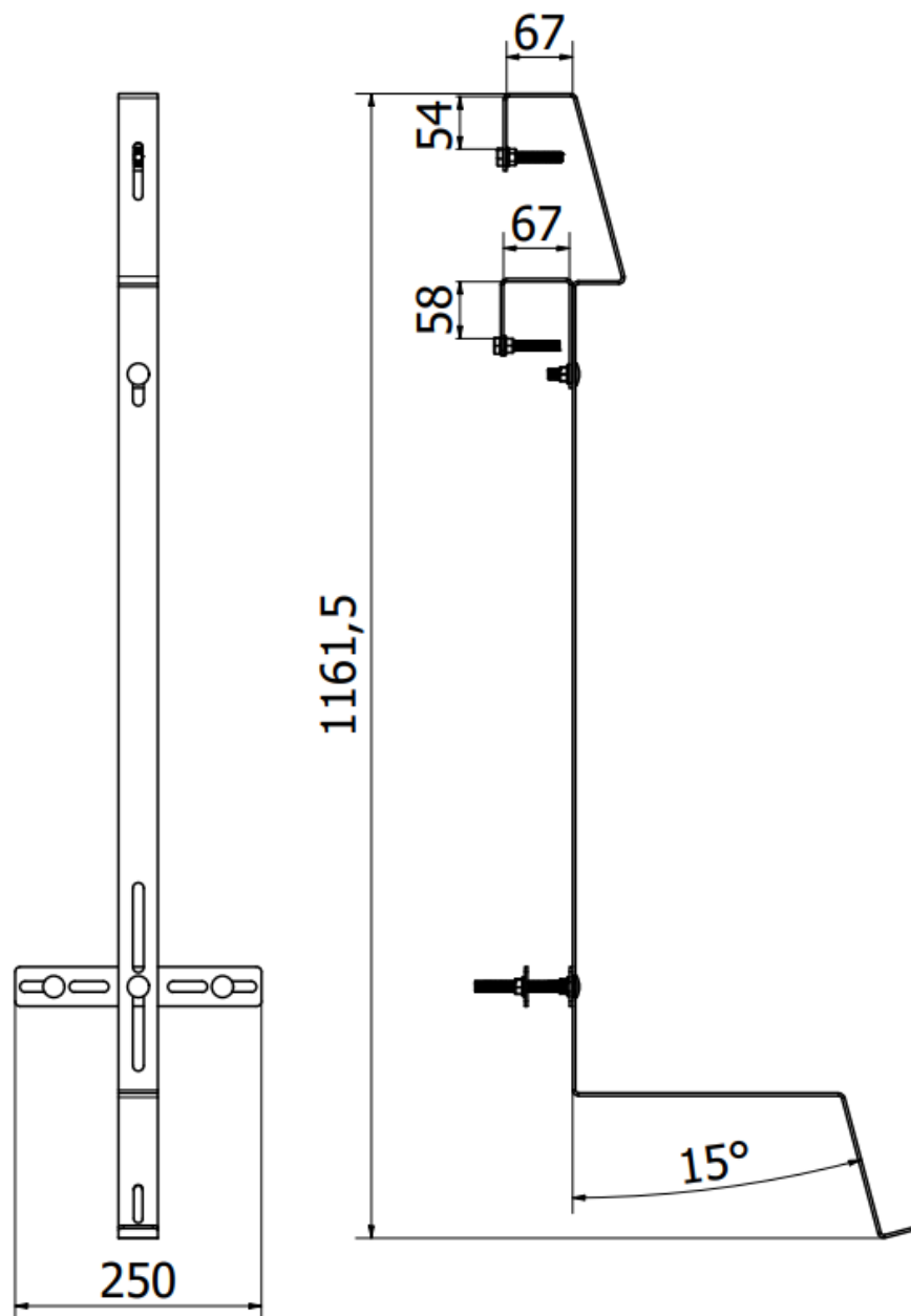
Rys.1 Wymiary konstrukcji
