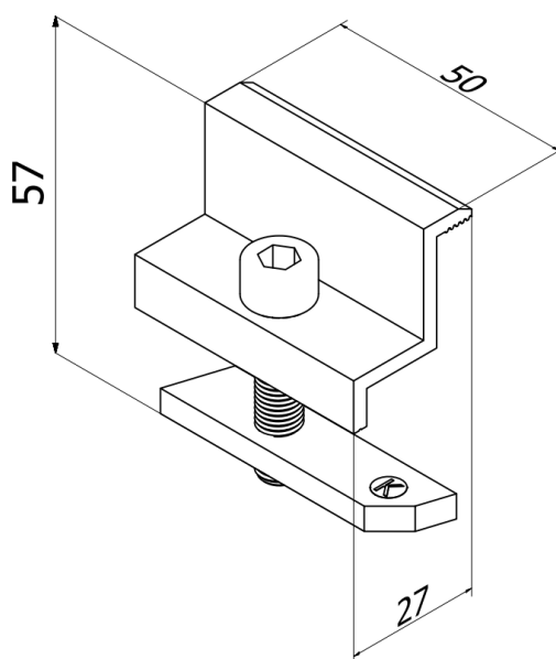
Rys.2 Wymiary elementu K-06-R
