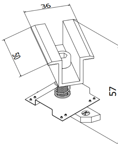
Rys.1 Wymiary elementu K-05-R
