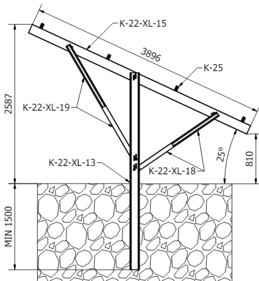
Rys.1 Wymiary konstrukcji
