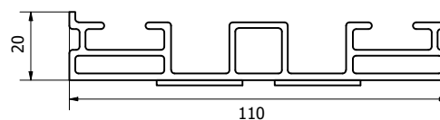
Rys.4 Szyna aluminiowa K-66-2
