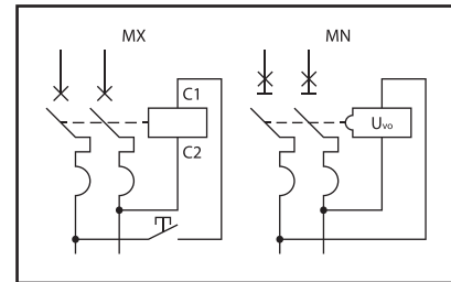
Schemat podłączenia Connection diagram
