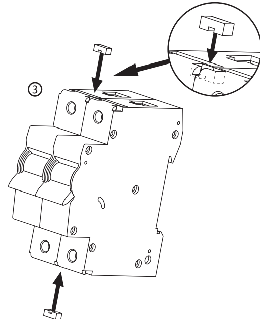
Schemat podłączenia Connection diagram
