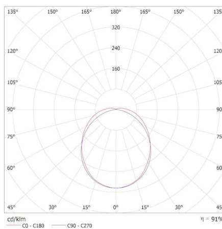
KANLUX S.A. (kat 38463) MAH MAX 19W 06 NW RYF / Krzywa rozsyłu światła (biegunowo)
